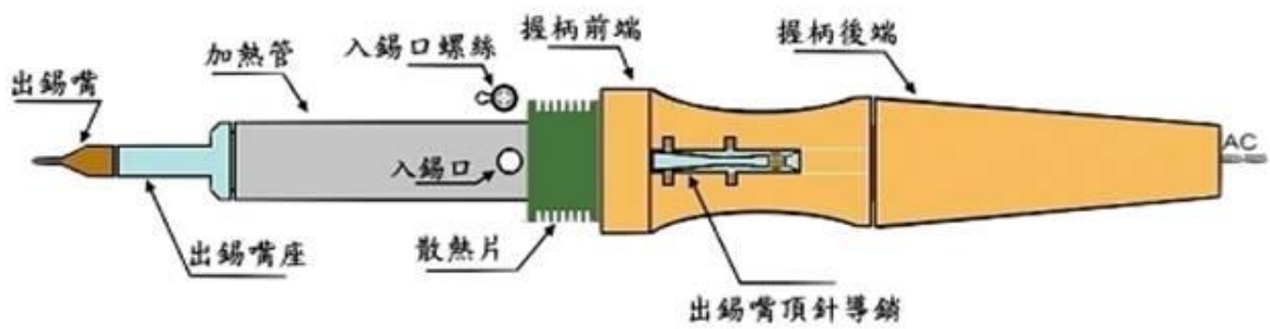
X-烙鐵 簡視圖
