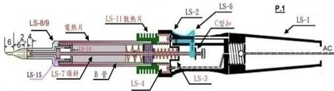
X-烙鐵 零件圖
